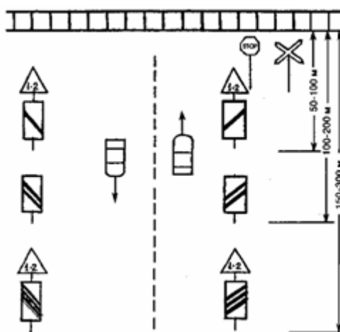
Рис. 88. Установка дорожных знаков перед железнодорожным переездом вне населенного пункта
